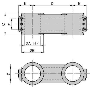
PARALLELO PARALLEL CLAMP MANCHON PARALLELE PARALLEL SOPORTE PARALELO
