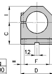
BASE BASE BLOC DE MONTAGE BLOCKHALTERUNG BASE
